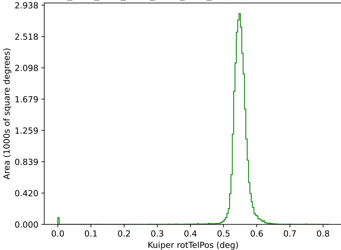
ddf_acor_sf15_ls30_lsr10_v3.4_10yrs g: Kuiper rotTelPos
