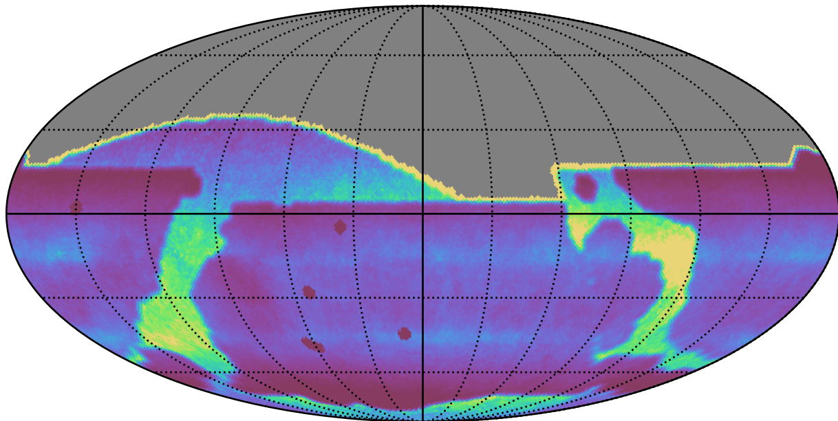
ddf_acor_sf15_lsf30_lsr10_v3.4_10yrs : DCRprecision
