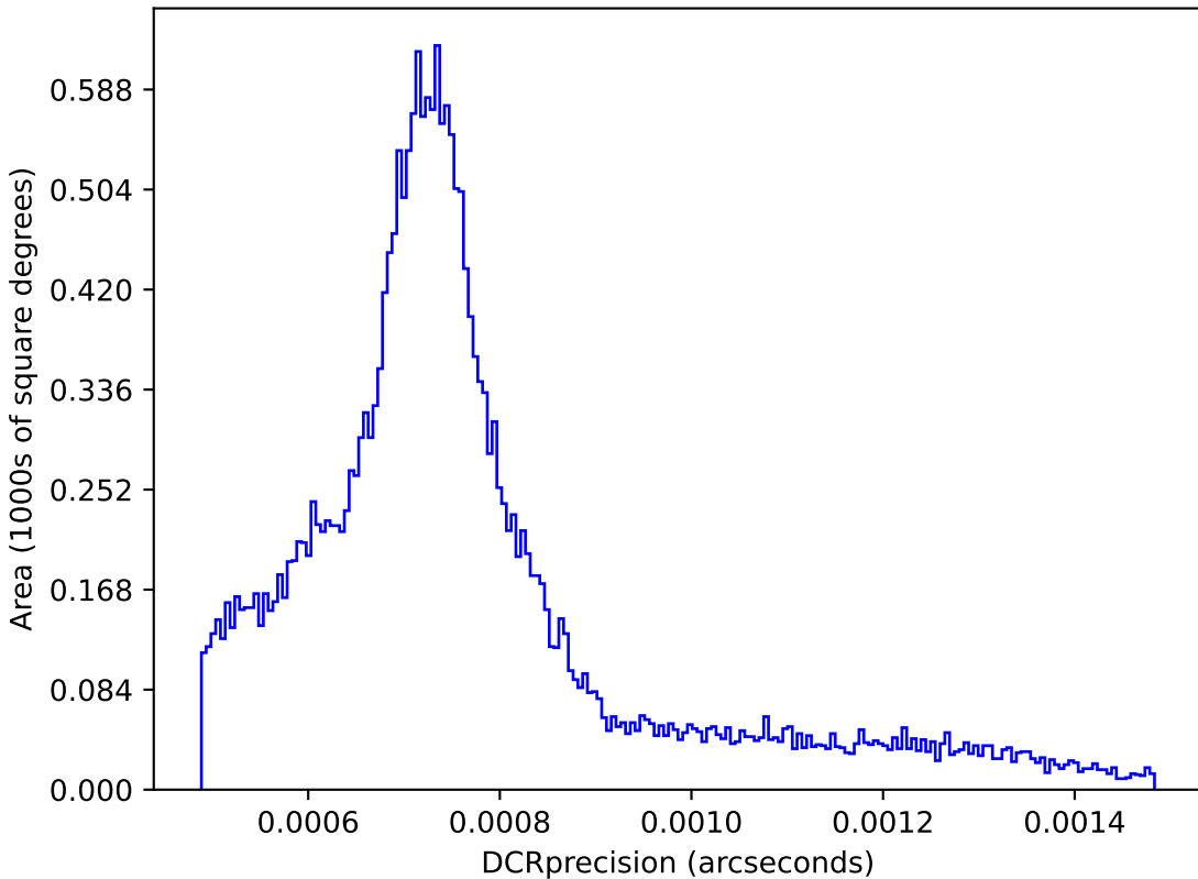
ddf_acor_sf15_lsf30_lsr10_v3.4_10yrs : DCRprecision
