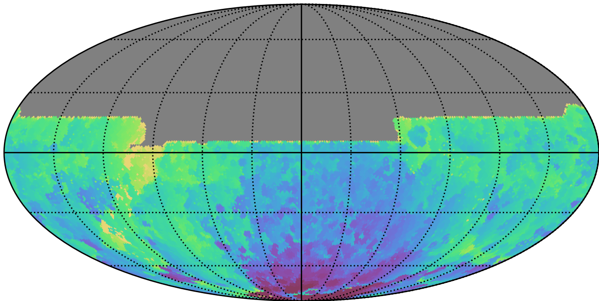
ddf_acor_sf15_lsf30_lsr10_v3.4_10yrs All sky y band: Min HA
