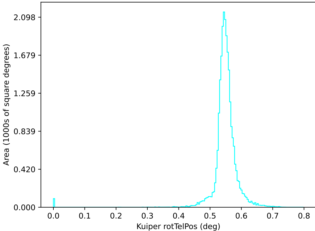
ddf_acor_sf15_ls20_lsr50_v3.4_10yrs u: Kuiper rotTelPos
