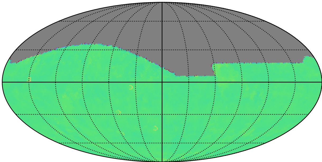
ddf_acor_sf15_lsf20_lsr50_v3.4_10yrs i: Kuiper rotTelPos
