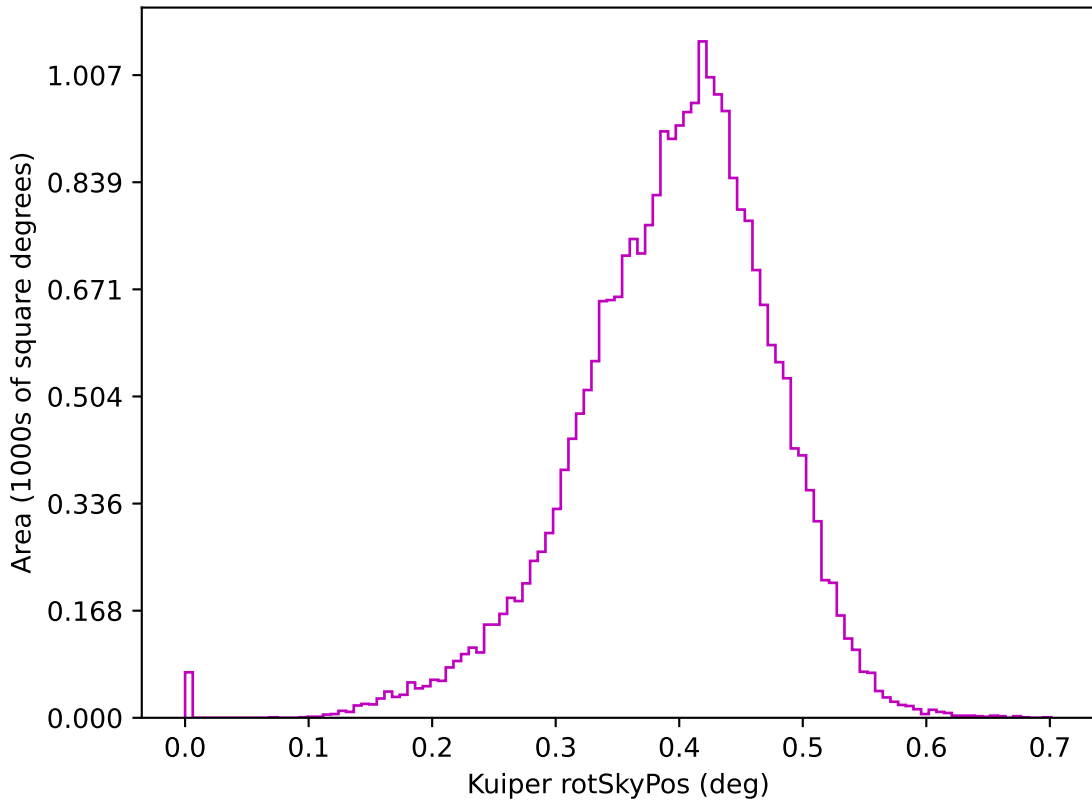
ddf_acor_sf15_lsf20_lsr50_v3.4_10yrs z: Kuiper rotSkyPos
