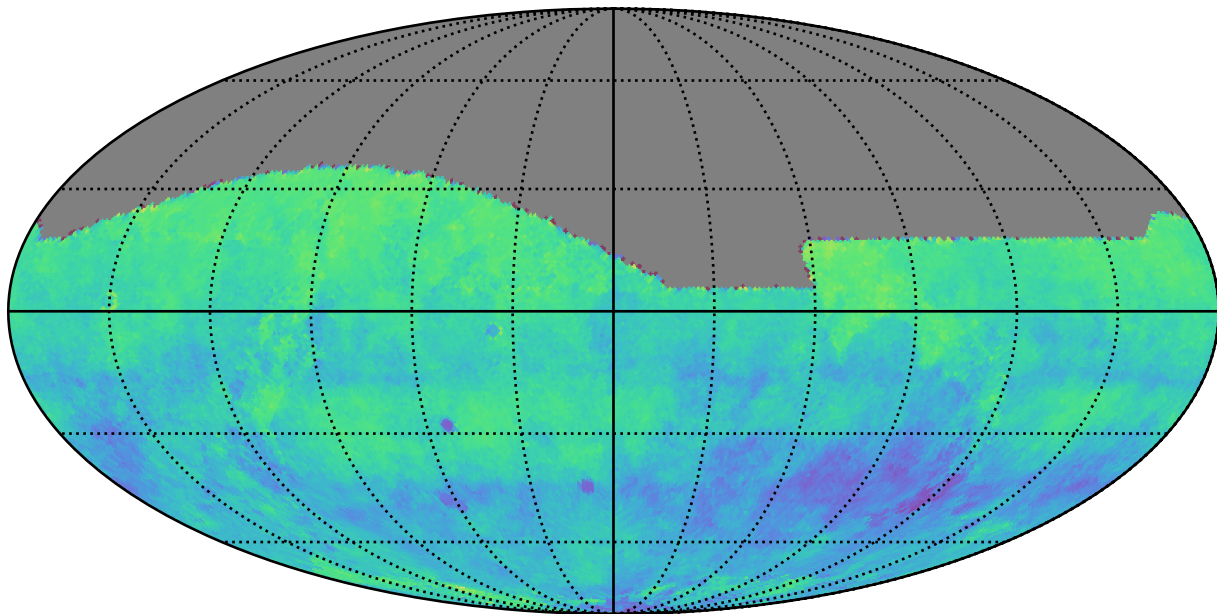
ddf_acor_sf15_lsf20_lsr50_v3.4_10yrs i: Kuiper rotSkyPos
