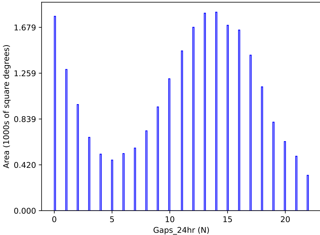
ddf_acor_sf15_lsf20_lsr50_v3.4_10yrs y band: Gaps_24hr
