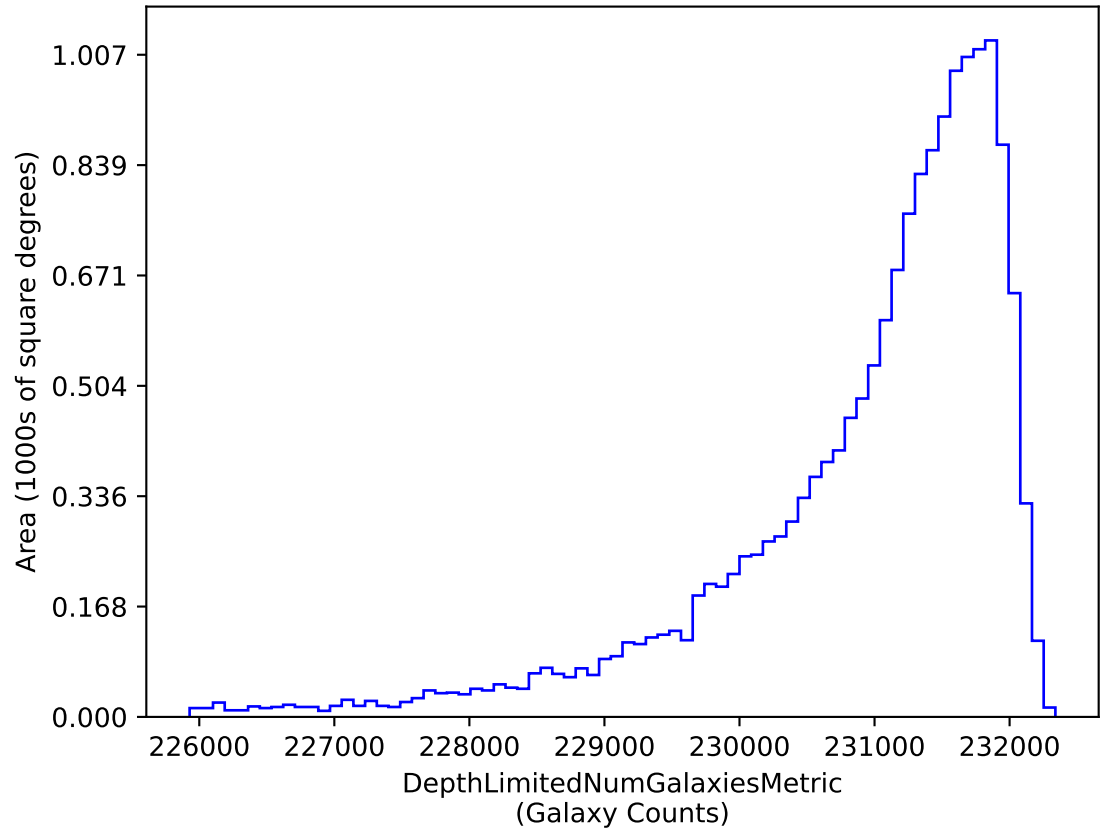
ddf_acor_sf15_lsf20_lsr50_v3.4_10yrs i band galaxies non-DD: DepthLimitedNumGalaxiesMetric
