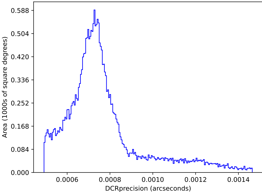
ddf_acor_sf15_lsf20_lsr50_v3.4_10yrs : DCRprecision
