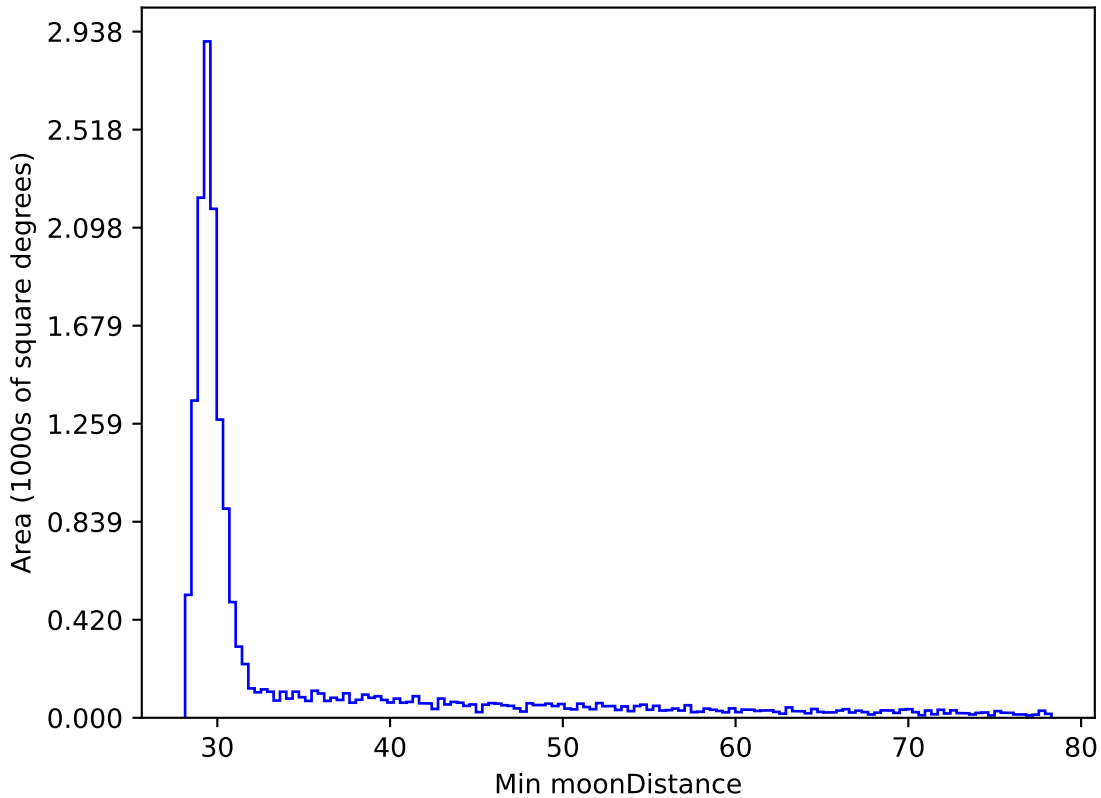
ddf_acor_sf15_lsf20_lsr50_v3.4_10yrs WFD y band: Min moonDistance
