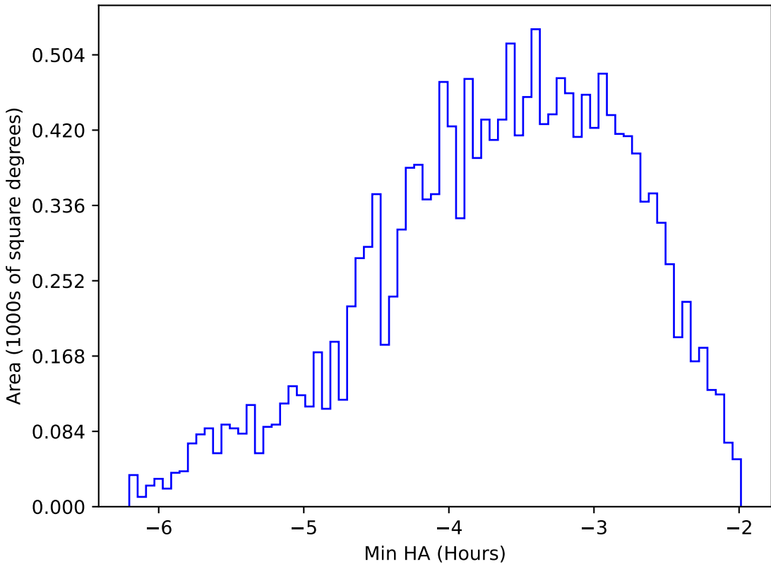
ddf_acor_sf15_lsf20_lsr50_v3.4_10yrs WFD y band: Min HA
