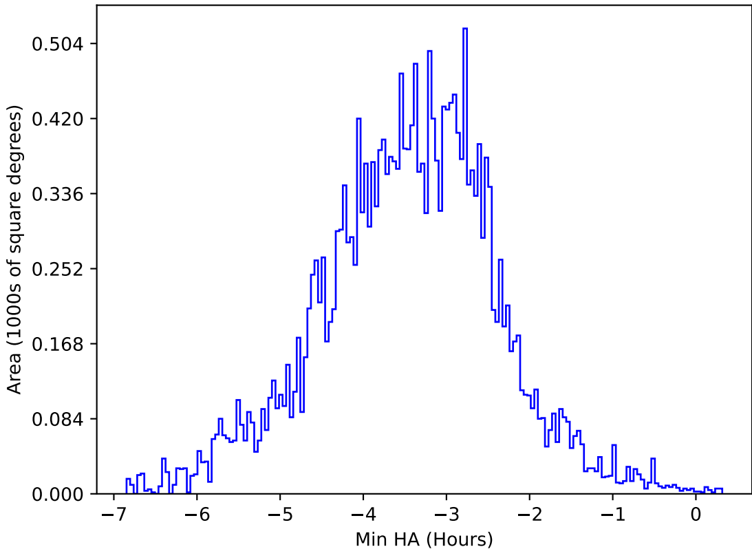
ddf_acor_sf15_lsf20_lsr50_v3.4_10yrs All sky y band: Min HA
