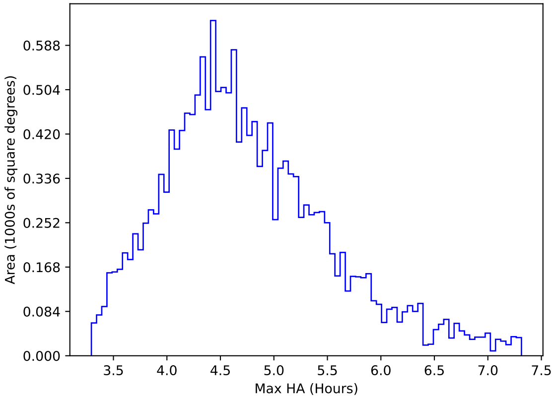
ddf_acor_sf15_lsf20_lsr50_v3.4_10yrs WFD y band: Max HA
