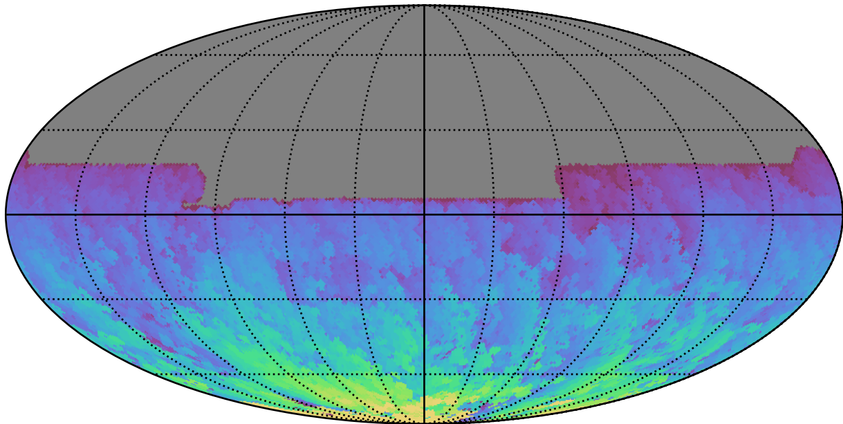
ddf_acor_sf15_lsf20_lsr50_v3.4_10yrs All sky y band: Max HA
