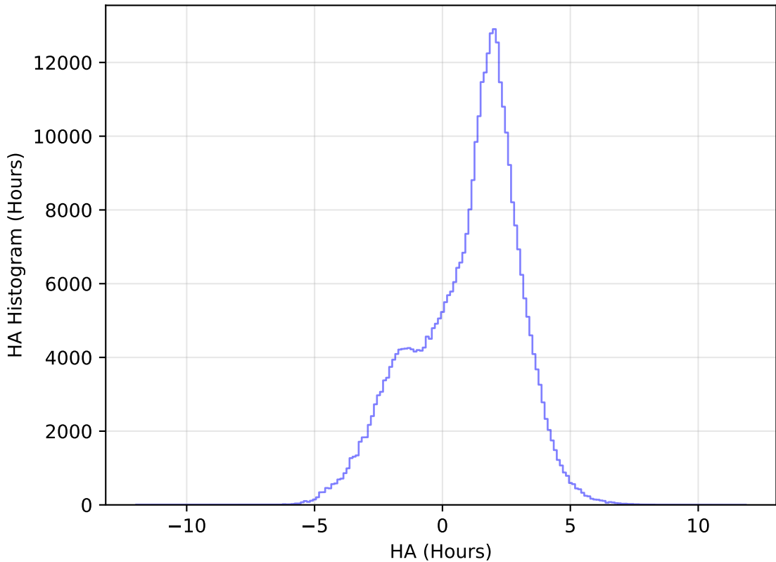
ddf_acor_sf15_lsf20_lsr50_v3.4_10yrs All sky y band: HA Histogram
