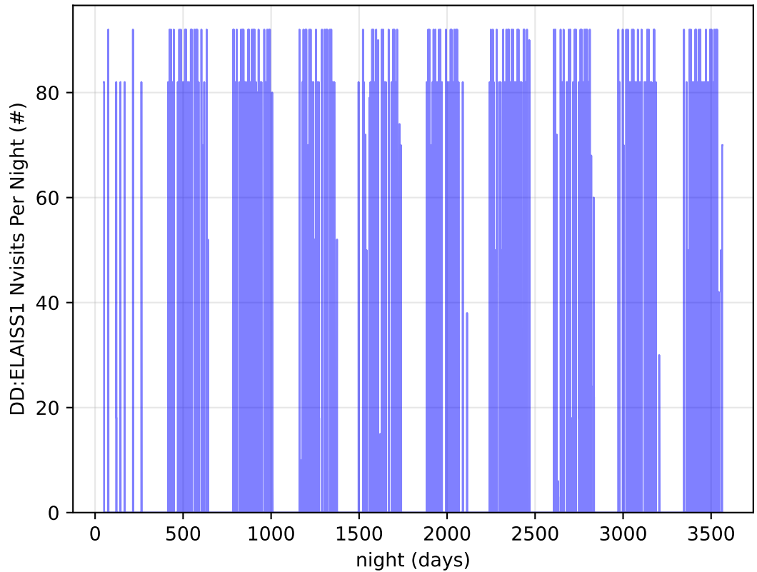
ddf_acor_sf15_lsf20_lsr50_v3.4_10yrs all bands: DD:ELAISS1 Nvisits Per Night
