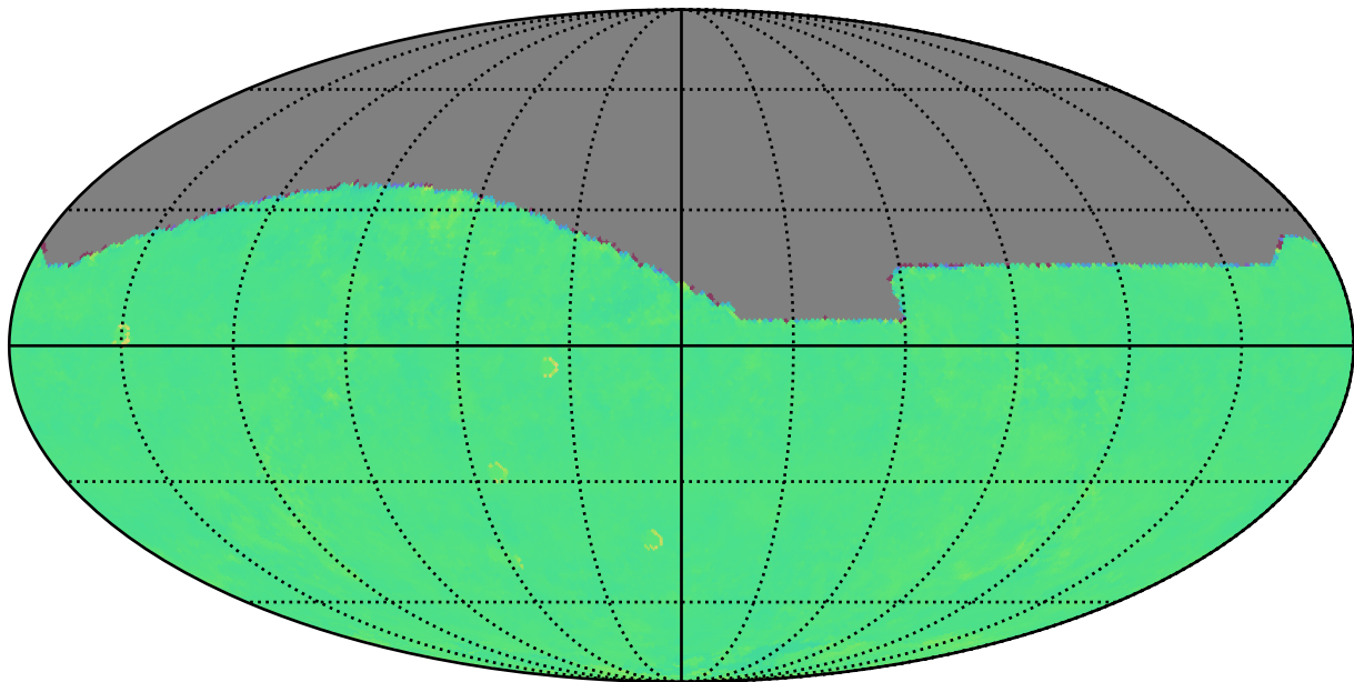
ddf_acor_sf15_lsf20_lsr20_v3.4_10yrs i: Kuiper rotTelPos
