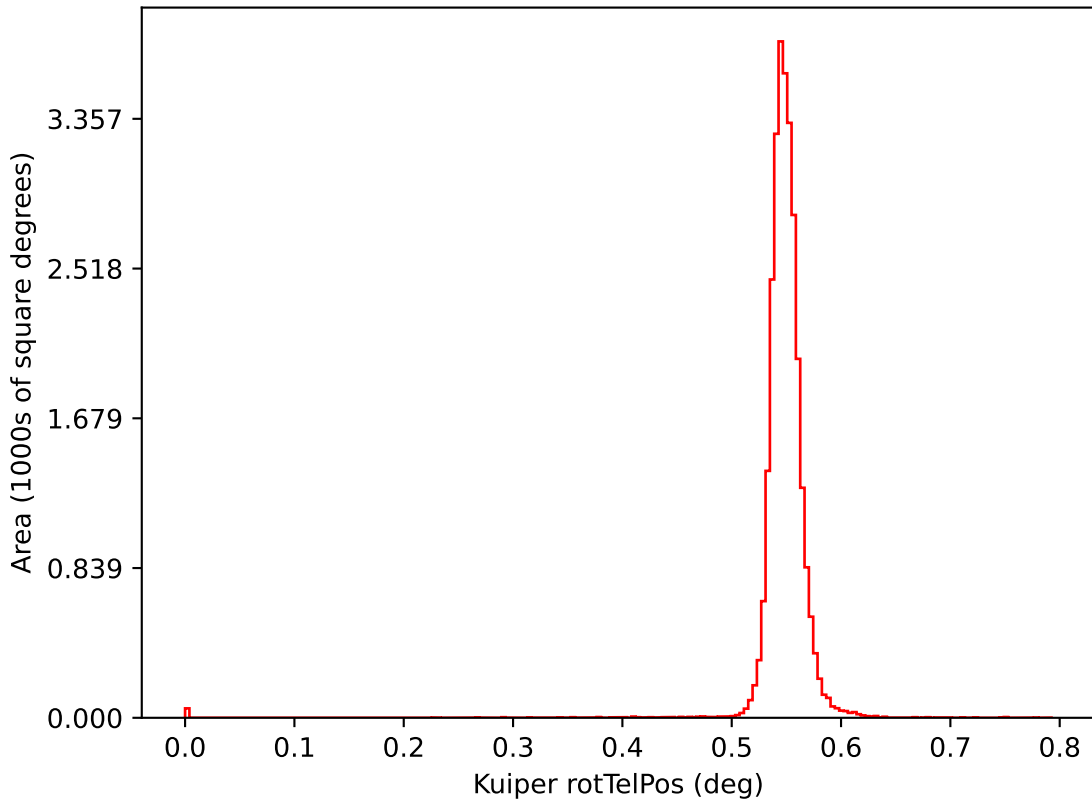
ddf_acor_sf15_lsf20_lsr20_v3.4_10yrs i: Kuiper rotTelPos
