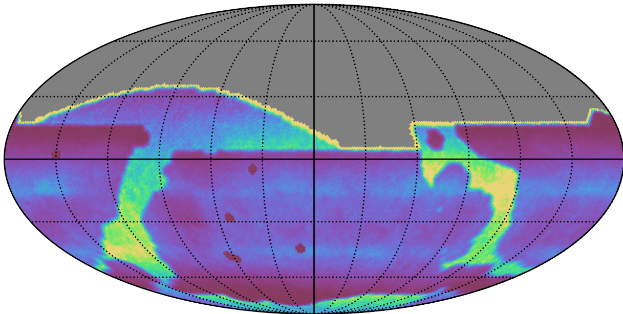
ddf_acor_sf15_lsf20_lsr20_v3.4_10yrs : DCRprecision
