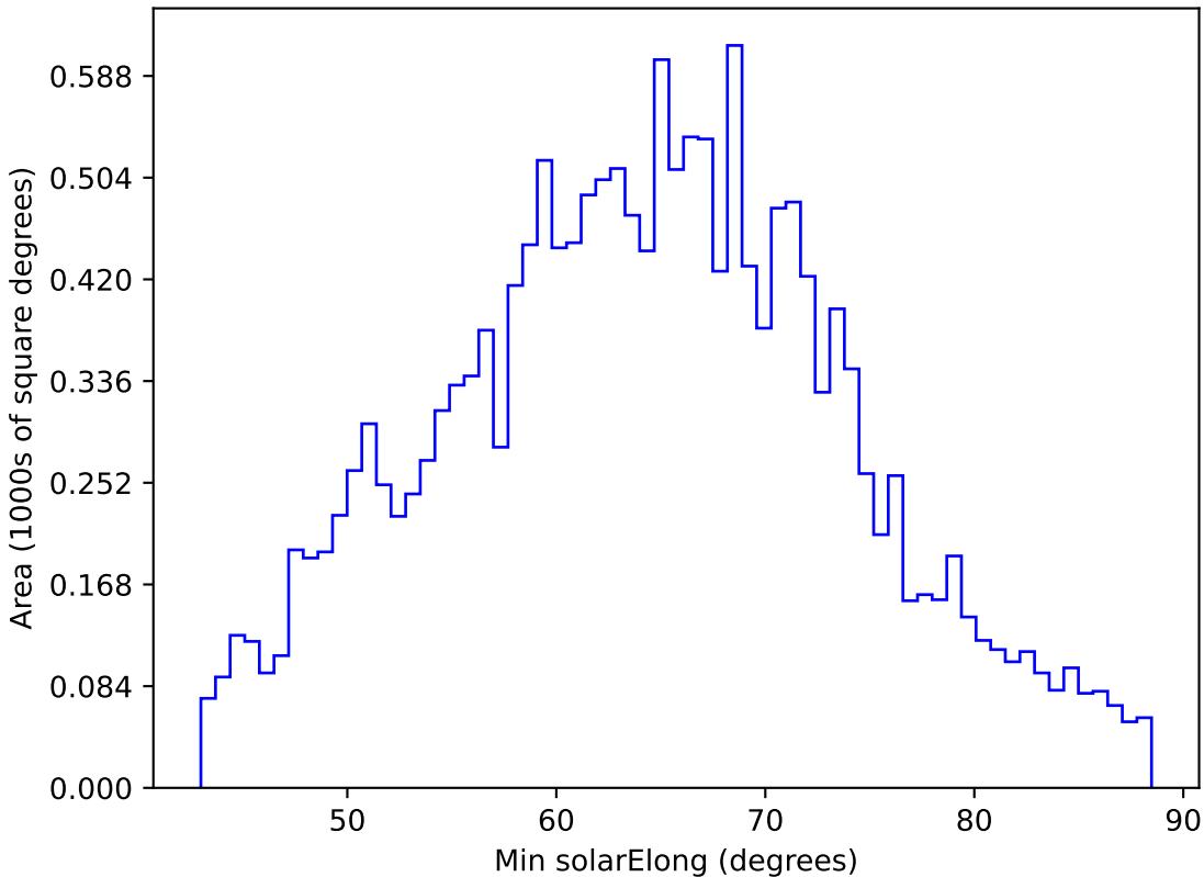
ddf_acor_sf15_lsf20_lsr20_v3.4_10yrs WFD y band: Min solarElong
