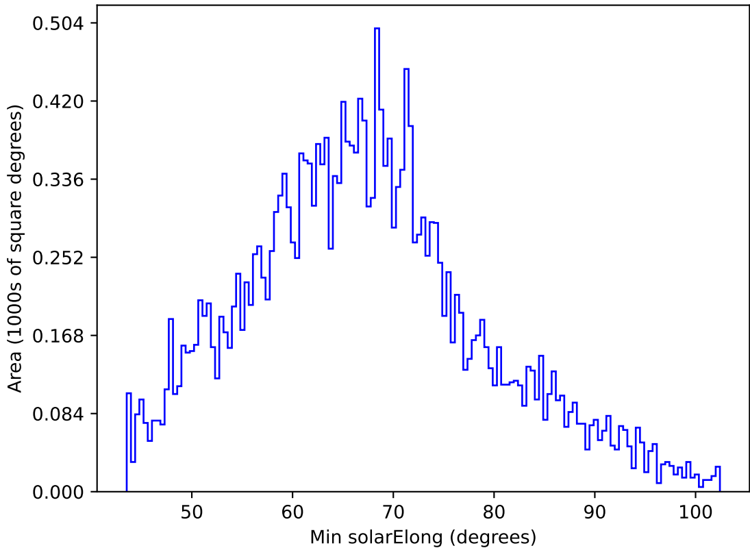
ddf_acor_sf15_lsf20_lsr20_v3.4_10yrs All sky y band: Min solarElong
