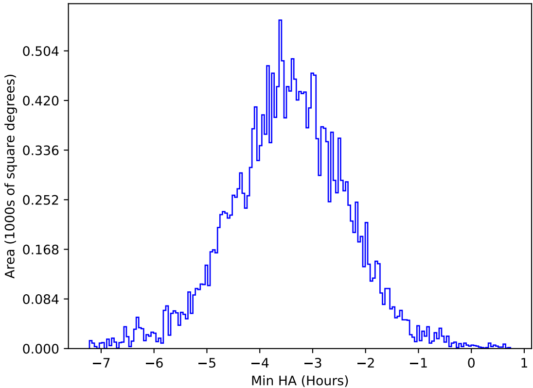
ddf_acor_sf15_lsf20_lsr20_v3.4_10yrs All sky y band: Min HA
