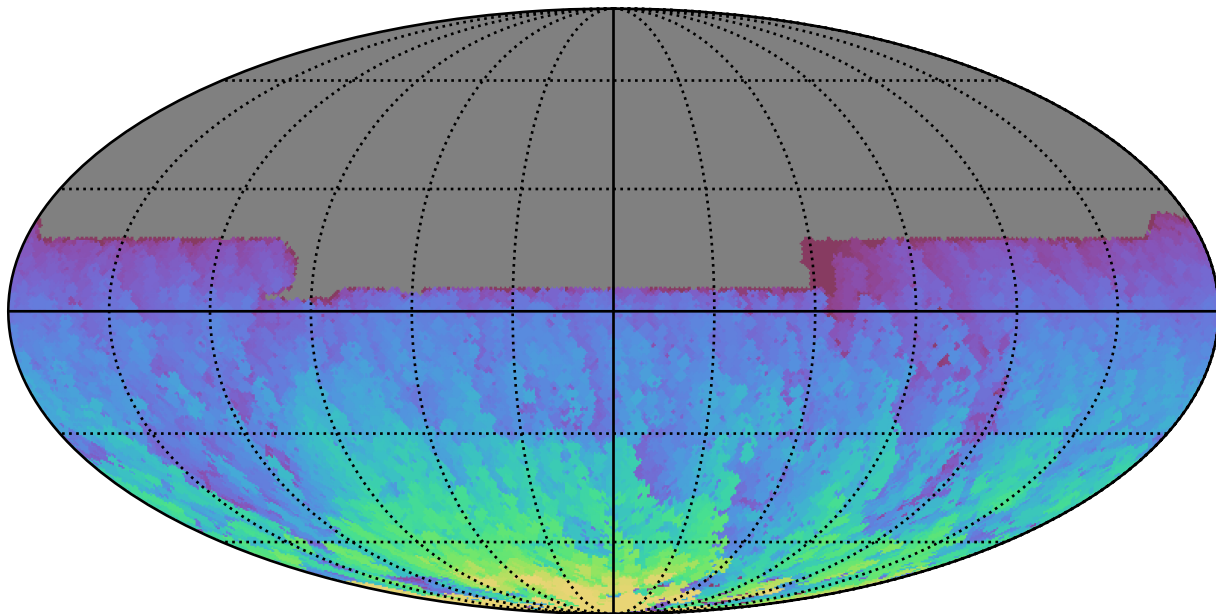
ddf_acor_sf15_lsf20_lsr20_v3.4_10yrs All sky y band: Max HA
