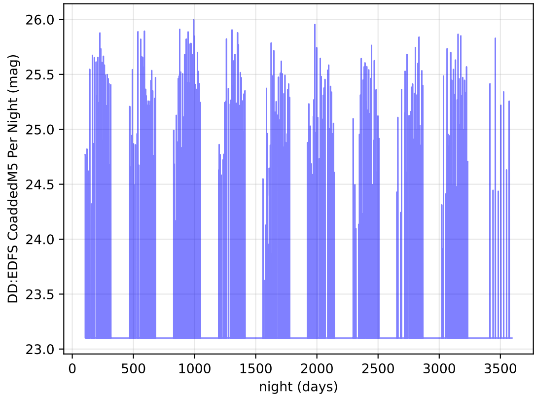
ddf_acor_sf15_Isf20_Isr20_v3.4_10yrs i band: DD:EDFS CoaddedM5 Per Night
