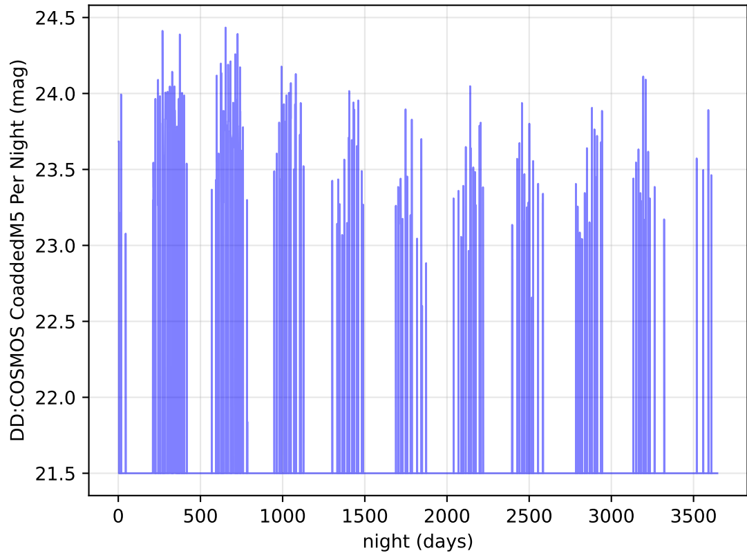
ddf_acor_sf15_lsf20_lsr20_v3.4_10yrs y band: DD:COSMOS CoaddedM5 Per Night
