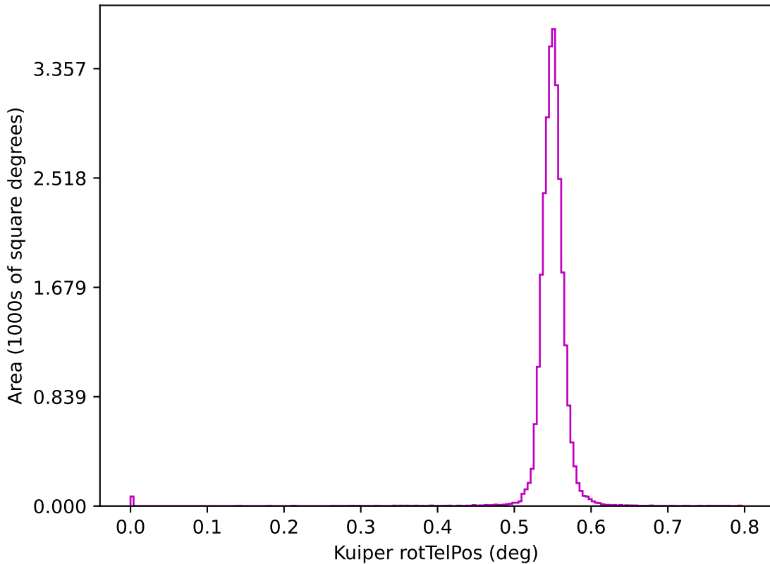
ddf_acor_sf15_lsf20_lsr10_v3.4_10yrs z: Kuiper rotTelPos
