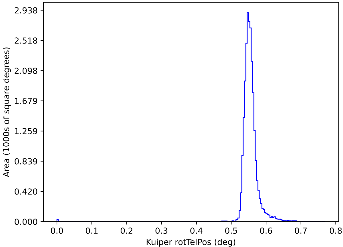
ddf_acor_sf15_lsf20_lsr10_v3.4_10yrs y: Kuiper rotTelPos
