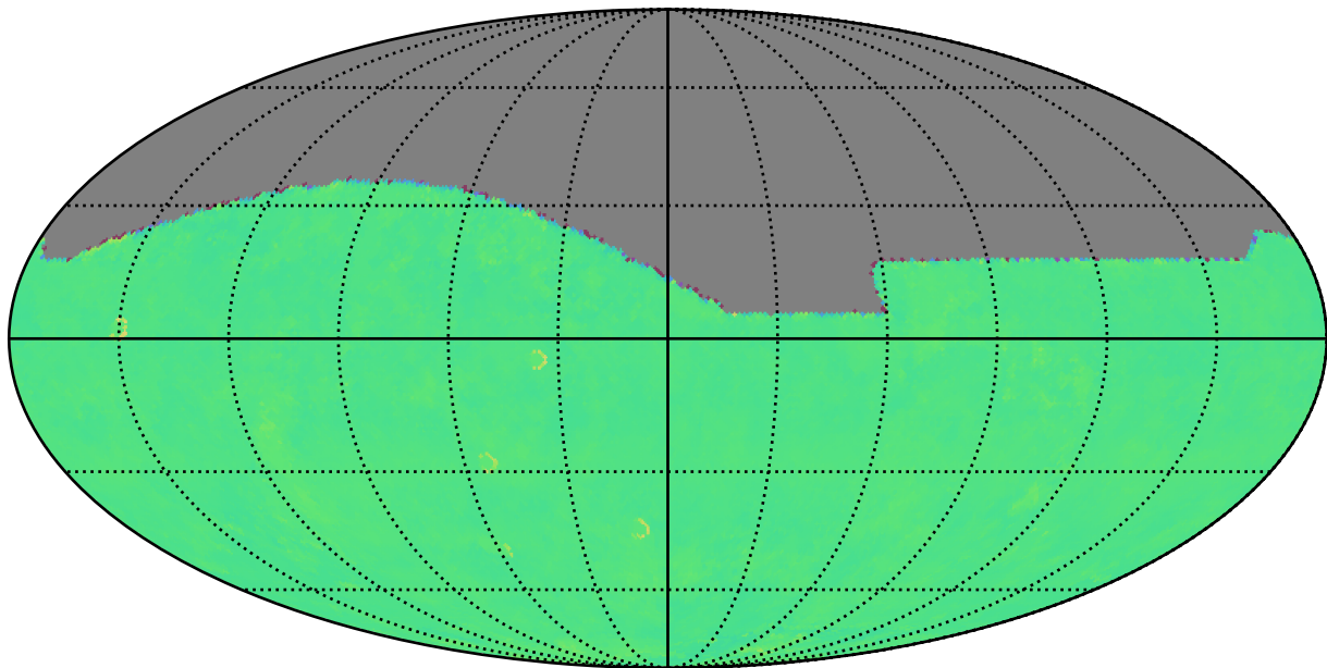
ddf_acor_sf15_lsf20_lsr10_v3.4_10yrs i: Kuiper rotTelPos
