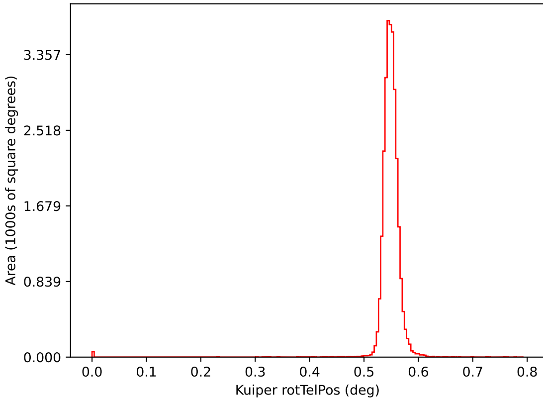
ddf_acor_sf15_lsf20_lsr10_v3.4_10yrs i: Kuiper rotTelPos
