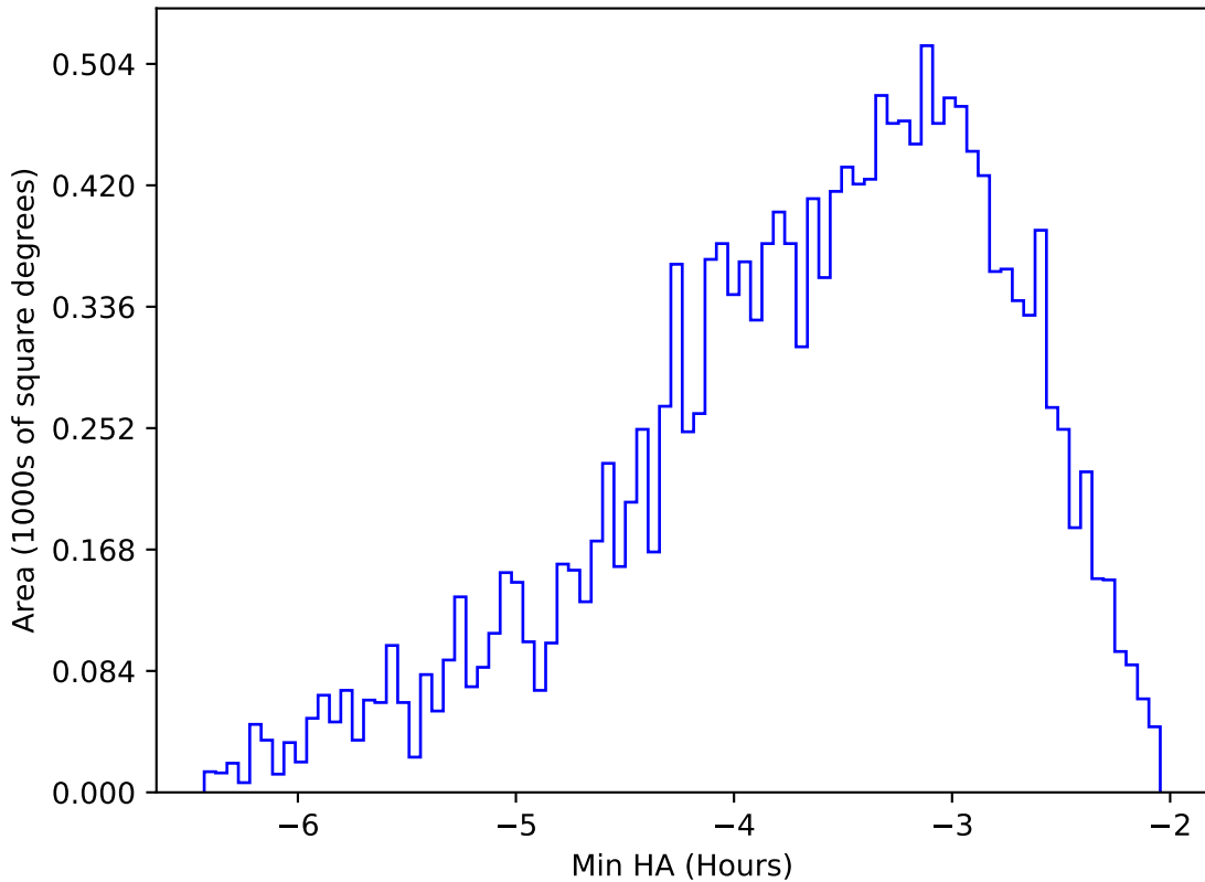
ddf_acor_sf15_lsf20_lsr10_v3.4_10yrs WFD y band: Min HA
