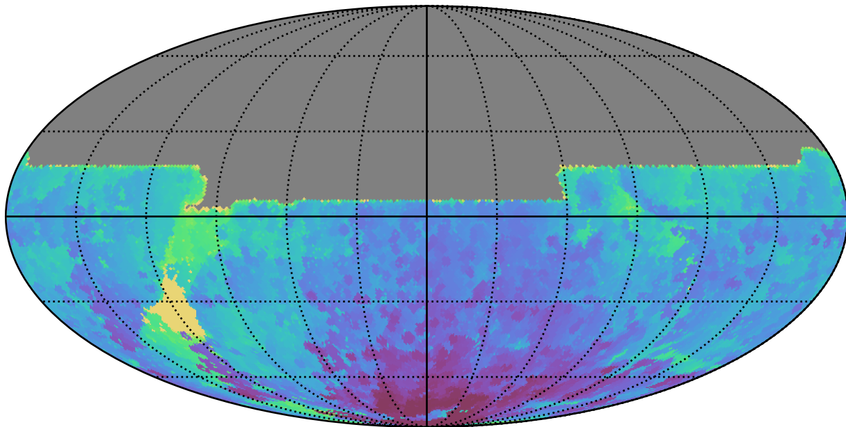
ddf_acor_sf15_lsf20_lsr10_v3.4_10yrs All sky y band: Min HA
