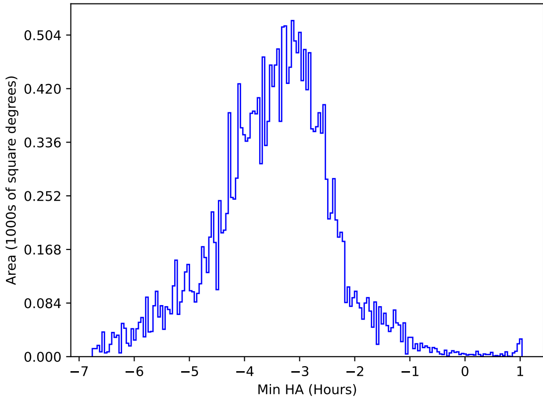
ddf_acor_sf15_lsf20_lsr10_v3.4_10yrs All sky y band: Min HA
