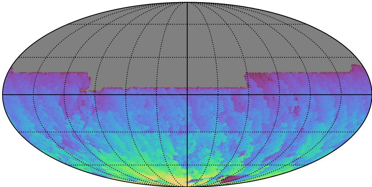
ddf_acor_sf15_lsf20_lsr10_v3.4_10yrs All sky y band: Max HA
