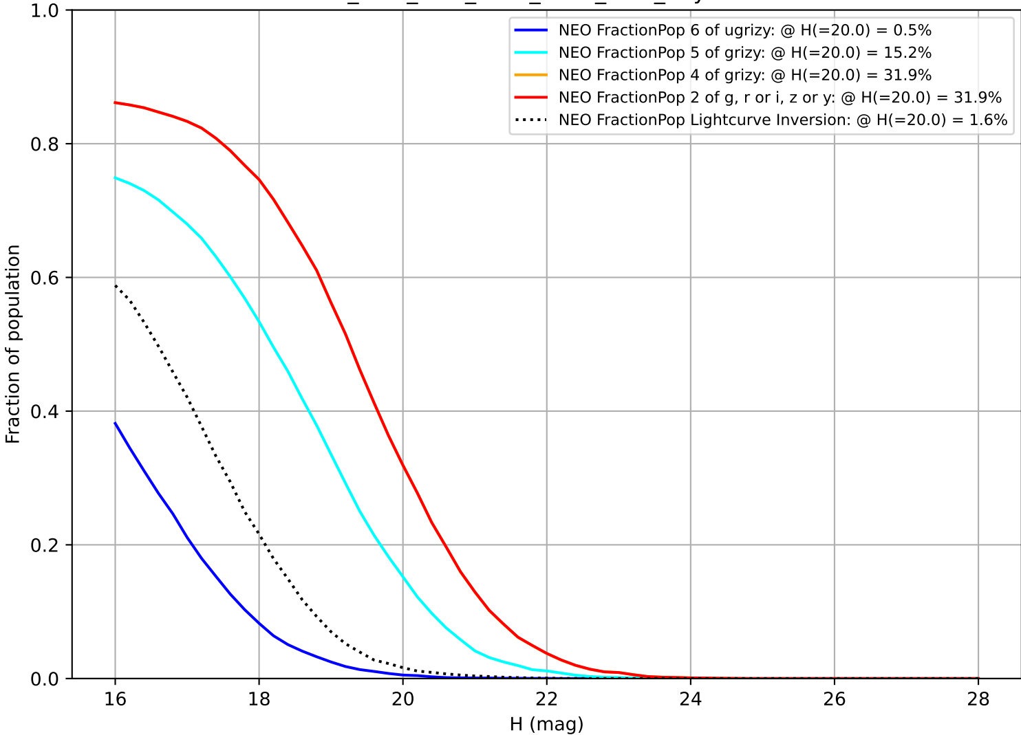
ddf_acor_sf10_lsf40_lsr50_v3.4_10yrs NEO
