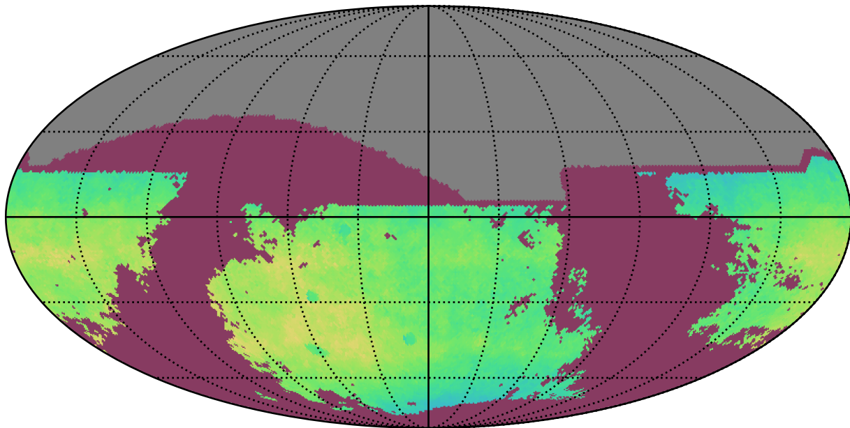
ddf_acor_sf10_lsf40_lsr50_v3.4_10yrs i: NgalScale
