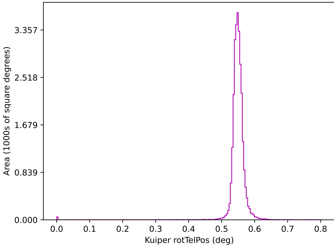
ddf_acor_sf10_lsf40_lsr50_v3.4_10yrs z: Kuiper rotTelPos
