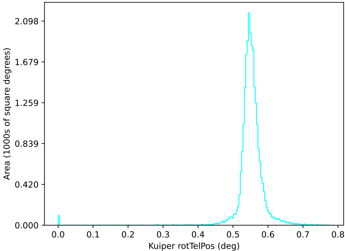
ddf_acor_sf10_ls40_lsr50_v3.4_10yrs u: Kuiper rotTelPos
