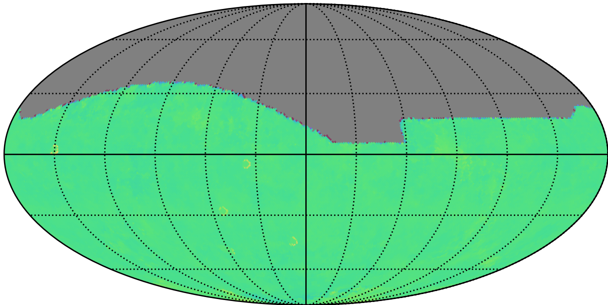
ddf_acor_sf10_lsf40_lsr50_v3.4_10yrs r: Kuiper rotTelPos
