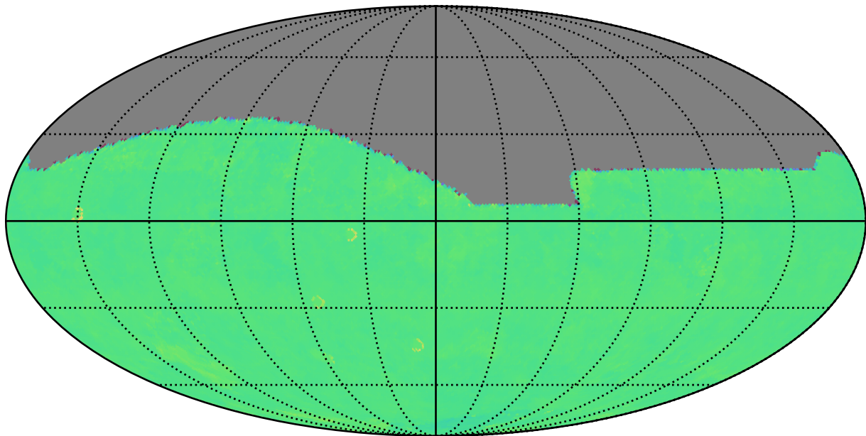
ddf_acor_sf10_lsf40_lsr50_v3.4_10yrs i: Kuiper rotTelPos
