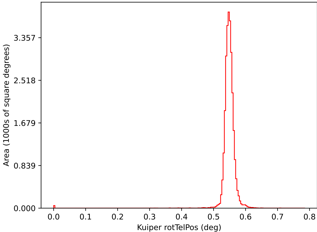
ddf_acor_sf10_lsf40_lsr50_v3.4_10yrs i: Kuiper rotTelPos
