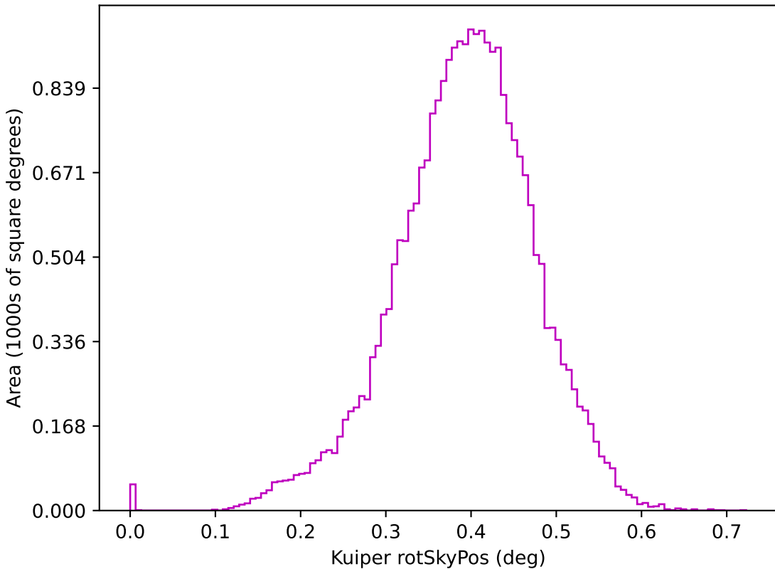
ddf_acor_sf10_lsf40_lsr50_v3.4_10yrs z: Kuiper rotSkyPos
