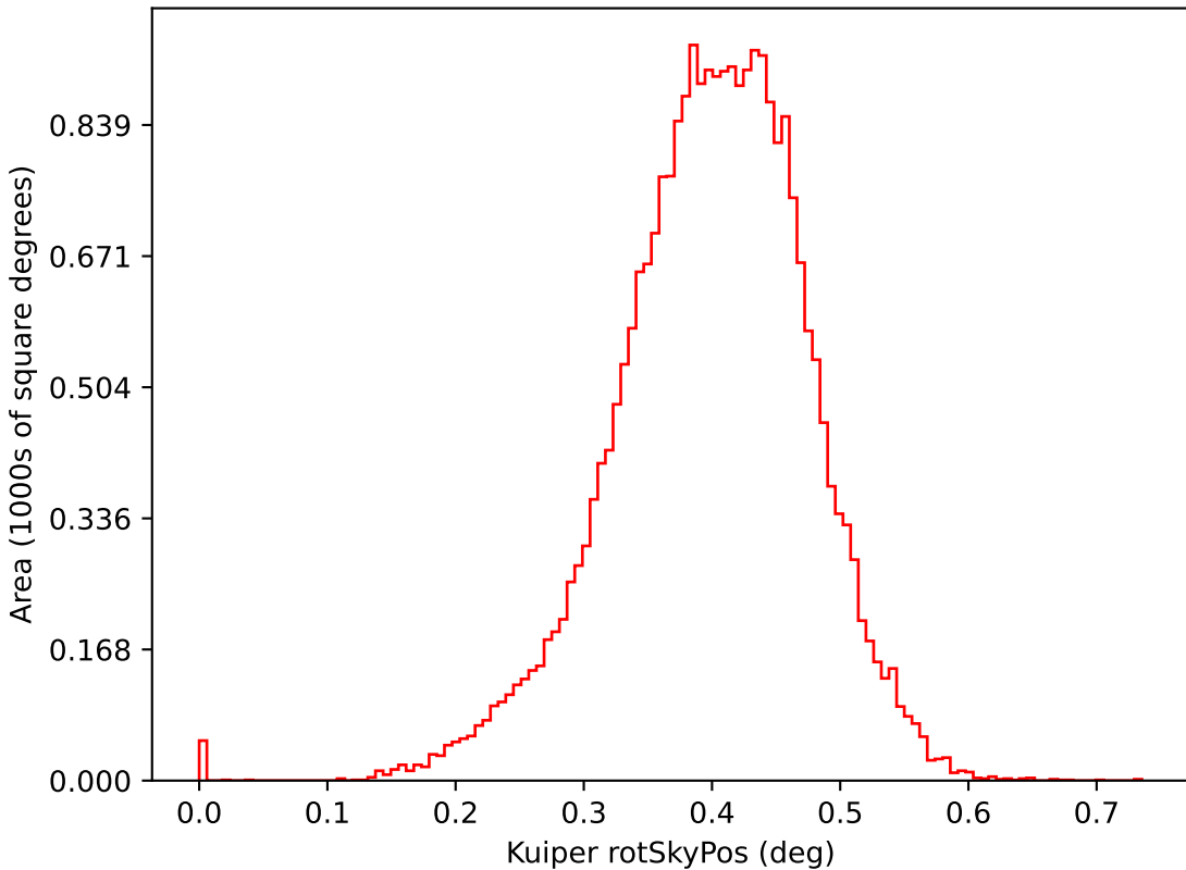
ddf_acor_sf10_ls40_lsr50_v3.4_10yrs i: Kuiper rotSkyPos
