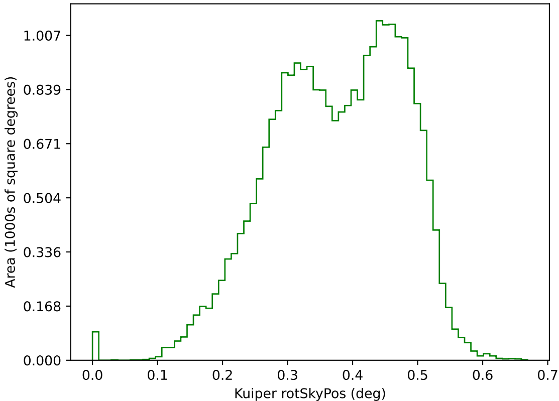
ddf_acor_sf10_lsf40_lsr50_v3.4_10yrs g: Kuiper rotSkyPos
