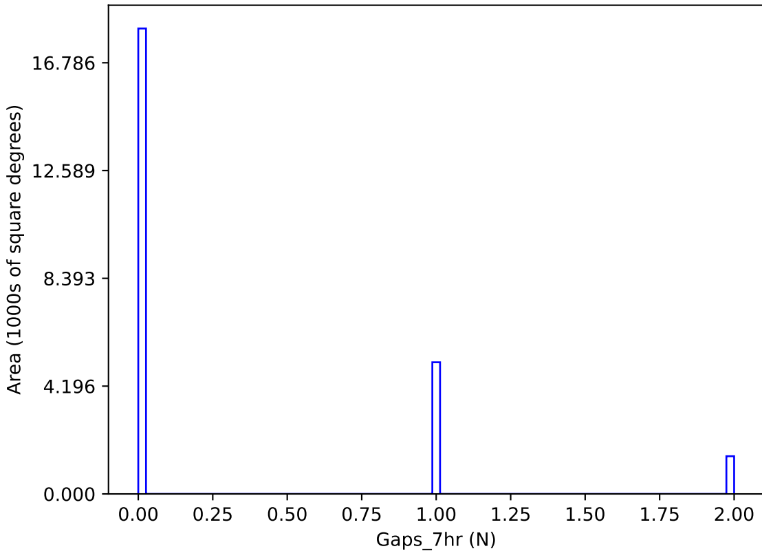
ddf_acor_sf10_lsf40_lsr50_v3.4_10yrs y band: Gaps_7hr
