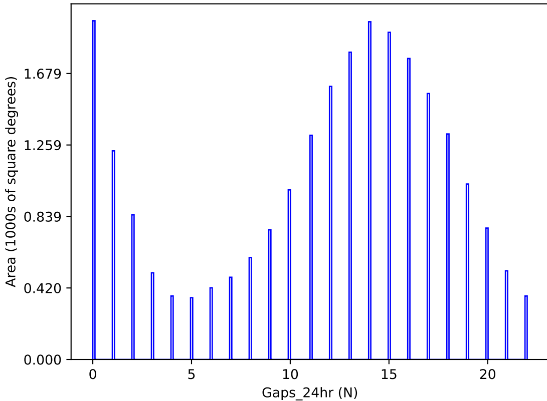
ddf_acor_sf10_lsf40_lsr50_v3.4_10yrs y band: Gaps_24hr
