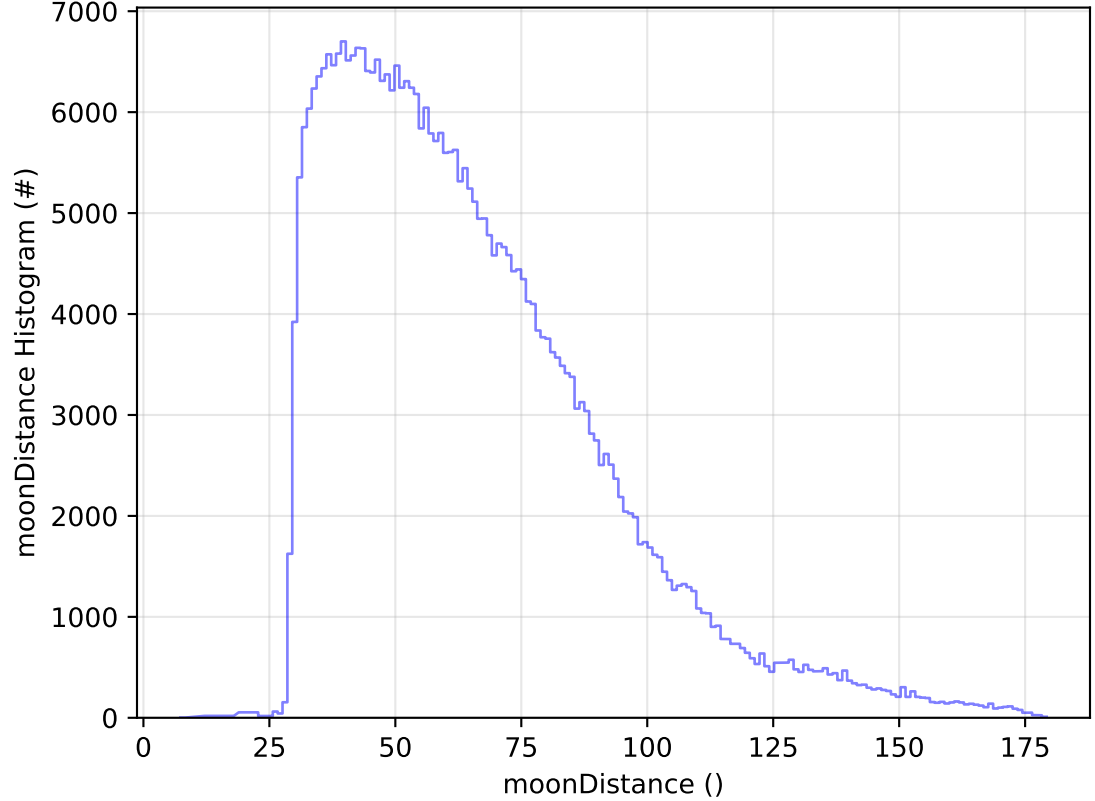
ddf_acor_sf10_lsf40_lsr50_v3.4_10yrs All sky y band: moonDistance Histogram
