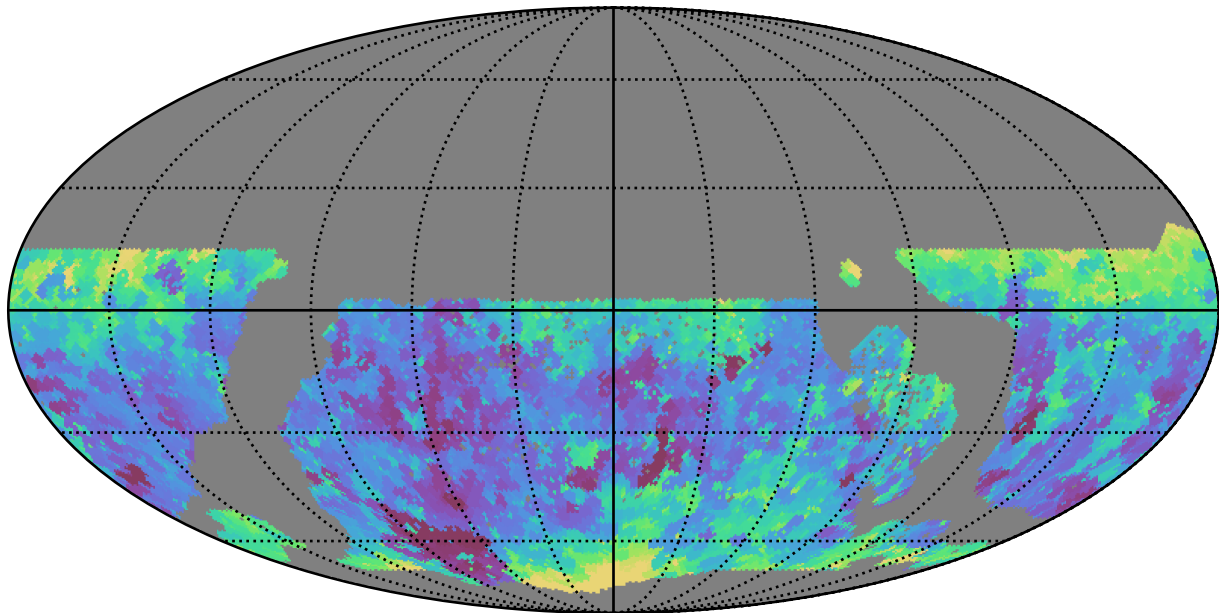
ddf_acor_sf10_lsf40_lsr50_v3.4_10yrs WFD y band: Min seeingEff
