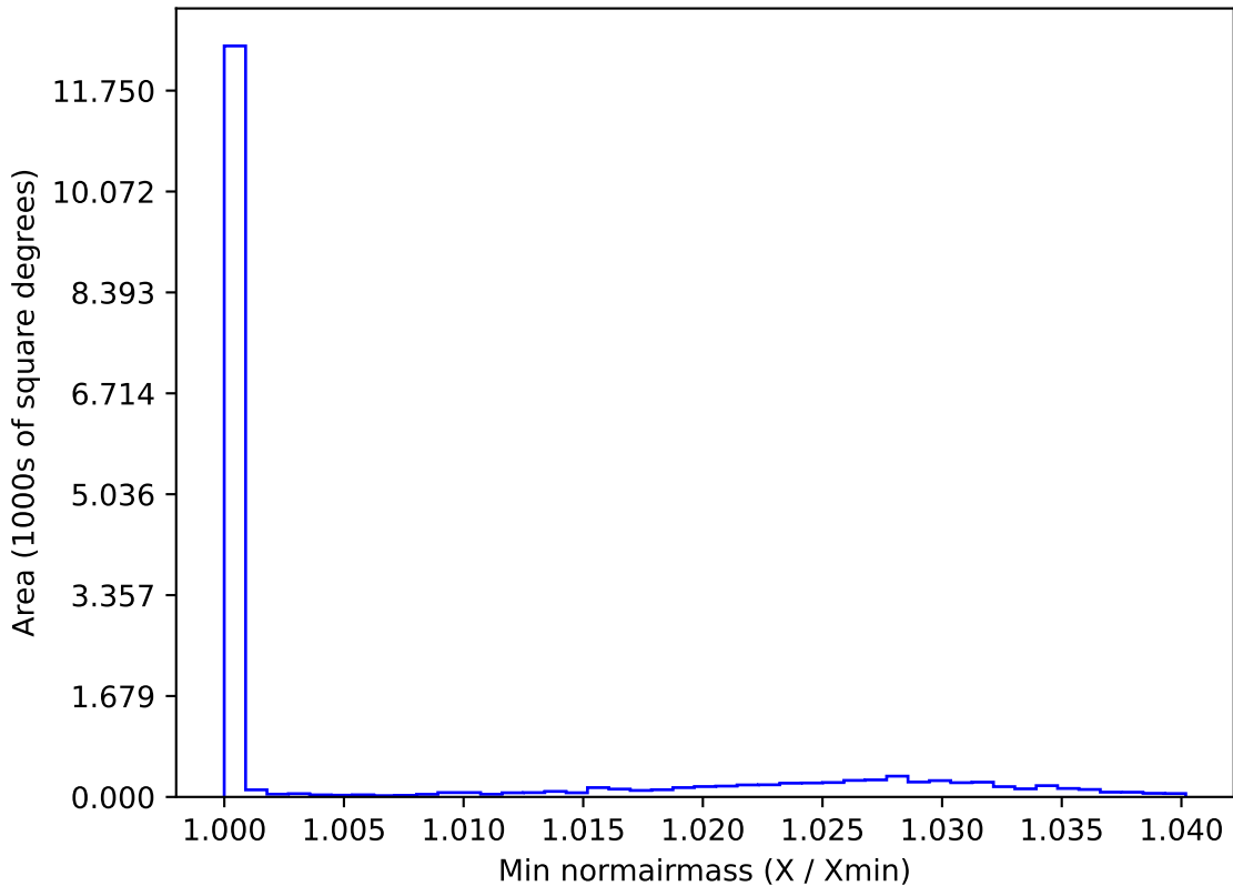
ddf_acor_sf10_lsf40_lsr50_v3.4_10yrs WFD y band: Min normairmass
